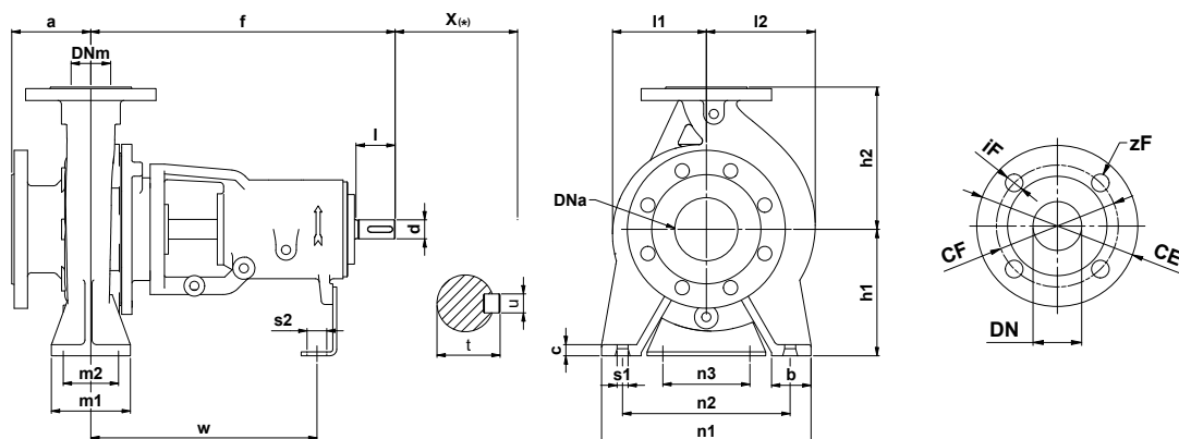
Dimensioni Flange Dimensions Flange EN1092-1 PN16
