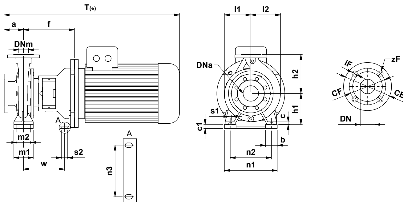
Dimensioni Flange Dimensions Flange EN1092-1 PN16
